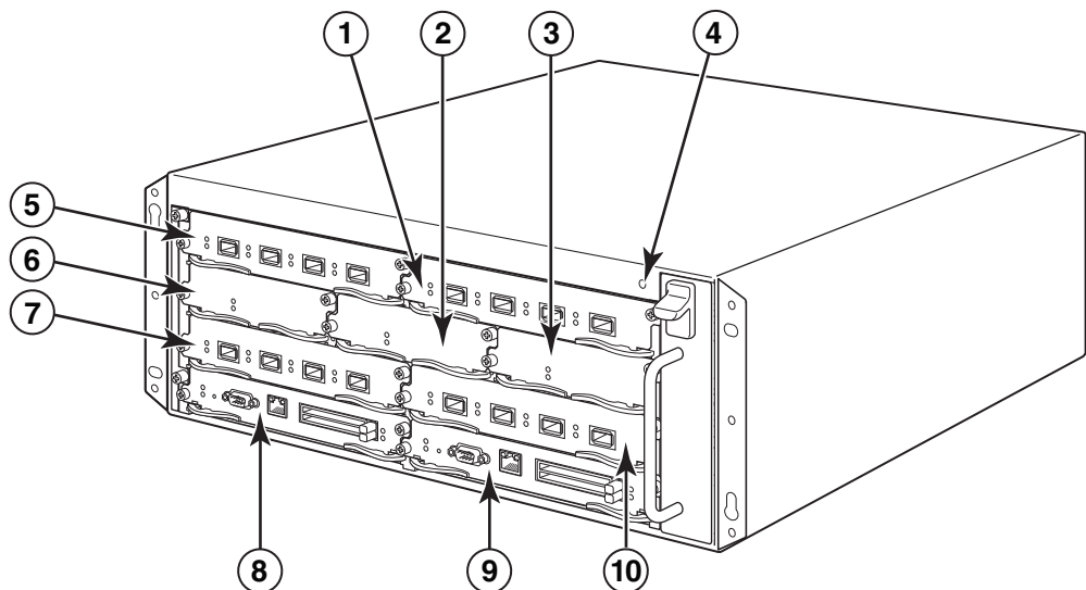
איור 1 תושבת PowerConnect B-MLXe Series בעלת 4 חריצים
